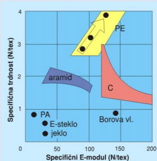
Specifična trdnost vlaken močno presega jeklo
